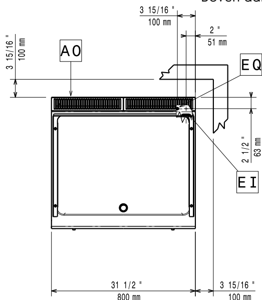
Boven aanzicht
